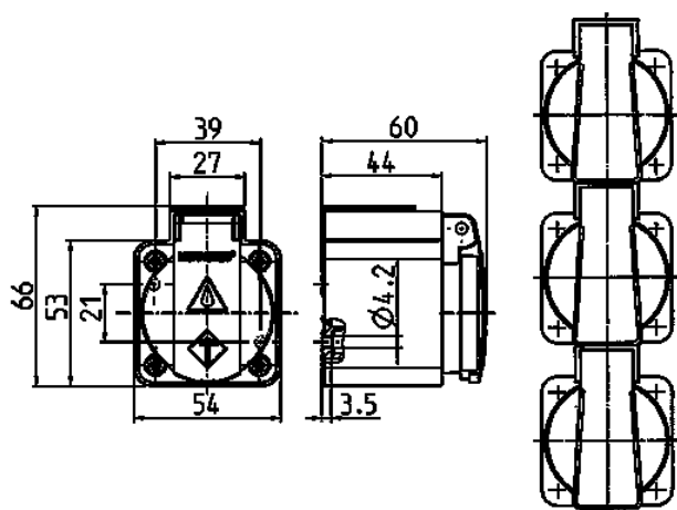
Tekening 1 MB 27/30
