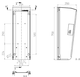
Schéma 1 MB 516 Dim. en mm
