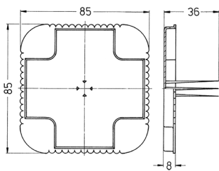
Schéma 1 MB 353 Dim. en mm
