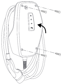
Fig. 15: Stenge produktet
