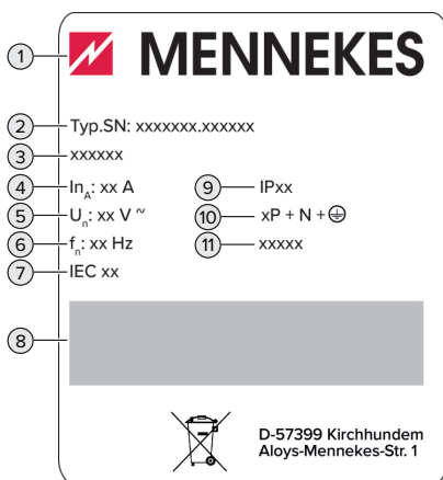
Fig. 1: Produkttypeskilt (eksempel)
