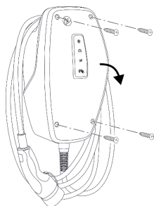
Pav. 5: Gaminį atidaryti
