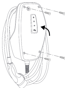
Obr. 15: Zavření výrobku
