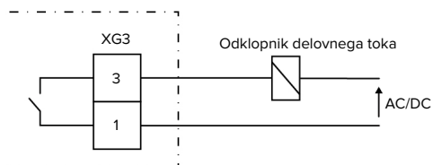
sl. 10: Osnovna vezalna shema: Prikluček zunanjega odklopnika delovnega toka
