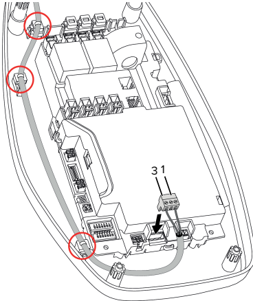
Kuva 9: Työvirtalaukaisijan liitännä
