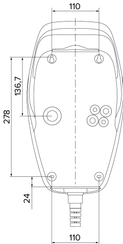
Fig. 6: Borrmått [mm]
