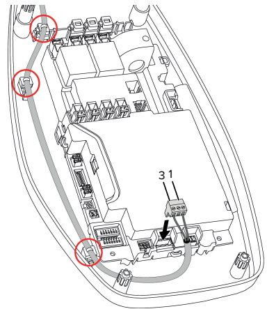
Afb. 9: Aansluiting arbeidsstroomactiveringsschakelaar
