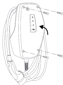
Fig. 15: Chiusura del prodotto
