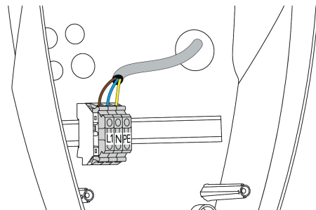
Fig. 8: Tilkobling spenningstilførsel
