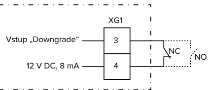
Obr. 14: Základní schéma zapojení: Připojení externího spínacího kontaktu (standardní nastavení: NO)
