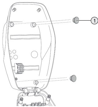
Pav. 7: Kamščiai
