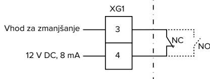
sl. 14: Osnovna vezalna shema: Priključitev zunanjega preklopnega kontakta (standardna nastavev: NO)
