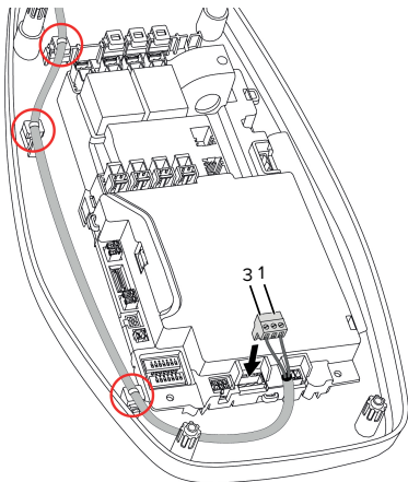
sl. 9: Prikluček odklopnika delovnega toka
