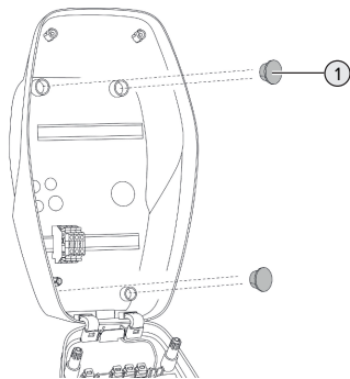
Obr. 7: Zátky
