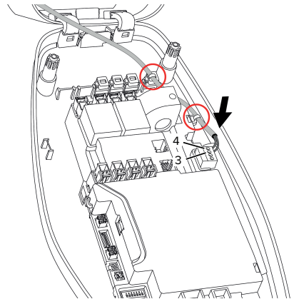
Fig. 13 : Raccordement de l'entrée Downgrade
