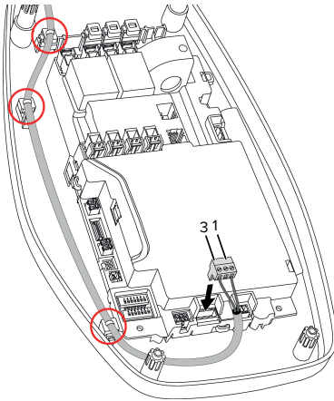
Fig. 9: Anslutning arbetsströmutlösare
