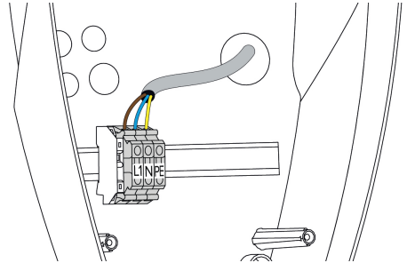
sl. 8: Priključek za oskrbo z napetostjo
