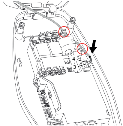
Obr. 13: Připojení vstupu Downgrade
