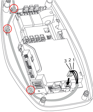
Şek. 11: Veri hattı bağlantısı [mm]
