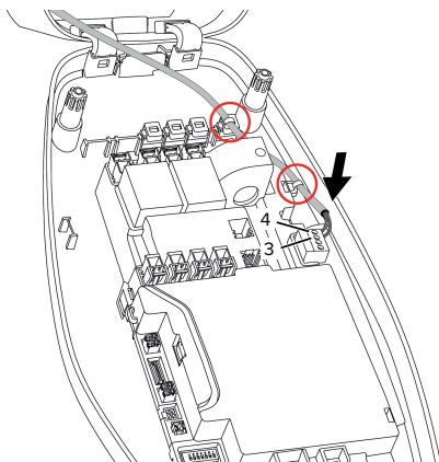
Fig. 13: Tilslutning downgrade-indgang
