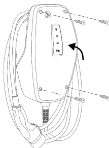
Εικ. 15: Κλείσιμο του προϊόντος
