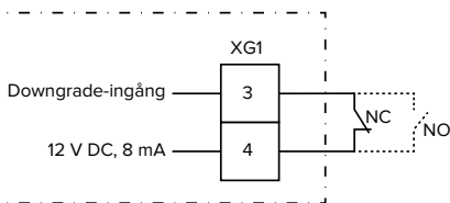
Fig. 14: Principkopplingsschema: Anslutning av en extern brytarkontakt (standardinställning: NO)
