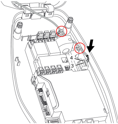
Şek. 13: Downgrade girişi bağlantısı
