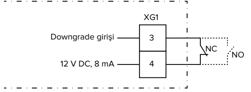
Şek. 14: Prensipsel devre şeması: Harici bir şalter kontaklarının bağlanması (standart ayar: NO)
