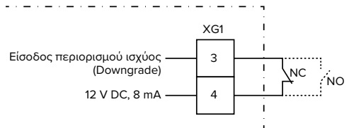
Εικ. 14: Διάγραμμα συνδεσμολογίας: Σύνδεση εξωτερικής επαφής μεταγωγής (βασική ρύθμιση: NO)
