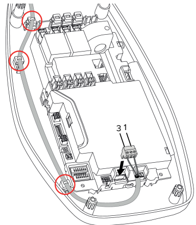
Εικ. 9: Σύνδεση ενεργοποιητή ρεύματος λειτουργίας
