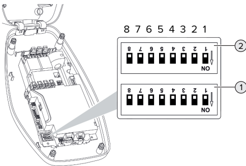
Abb. 12: DIP-Schalter (Auslieferungszustand)
