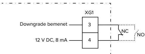
14. Ábra: Elvi kapcsolási rajz: Külső kapcsolóérintkező csatlakoztatása (normál beállítás: NO)
