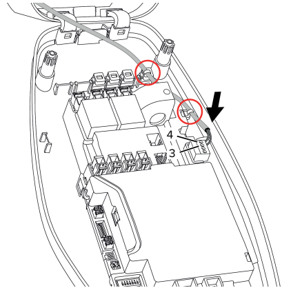
Abb. 13: Anschluss Downgrade-Eingang
