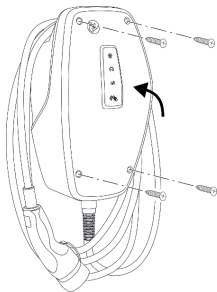
Fig. 15: Cierre del producto
