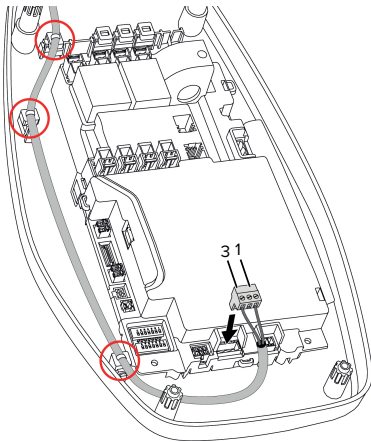
Abb. 9: Anschluss Arbeitsstromauslöser
