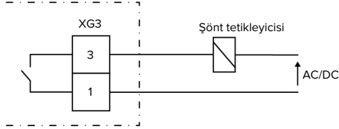
Şek. 10: Prensipsel devre şeması: Harici bir şönt tetikleyicisinin bağlantısı
