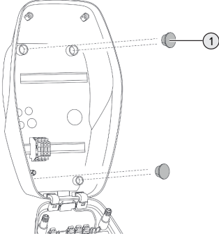
7. Ábra: Záródugók
