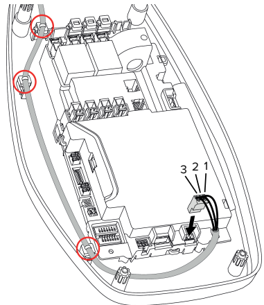
Afb. 11: Aansluiting dataleiding [mm]
