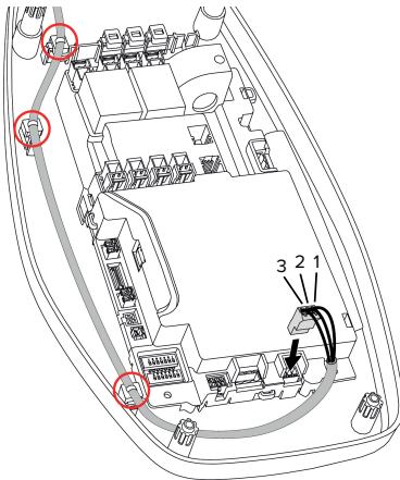
Abb. 11: Anschluss Datenleitung [mm]
