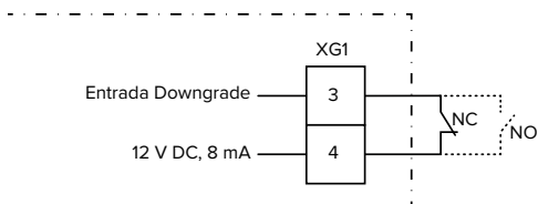
Fig. 14: Esquema de principio: Conexión de un contacto de conmutación externo (ajuste estándar: NO)
