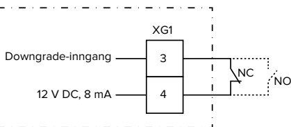
Fig. 14: Prinsipielt koblingsskjema: tilkobling av en ekstern bryterkontakt (standardinnstilling: NO)
