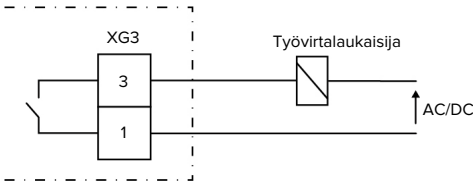
Kuva 10: Periaatekytkentäkaavio: ulkoisen työvirrän laukaisijan liitännä
