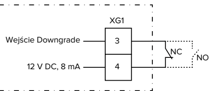
Ilustr. 14: Schemat blokowy: podłączenie zewnętrznego styku przełączającego (ustawienie standardowe: NO)
