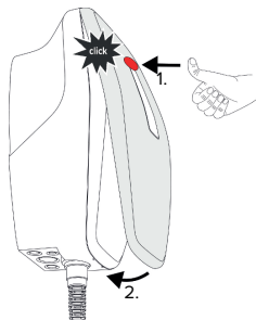
Fig. 17: Montaggio della cover anteriore - 1
