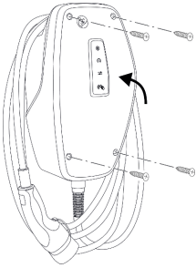
Kuva 15: Tuotteen sulkeminen
