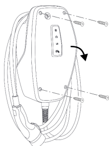
Fig. 5: Öppna produkten
