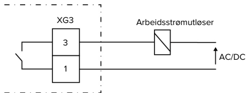
Fig. 10: Prinsipielt koblings skjema: Tilkobling av en ekstern arbeidsstrømutløser
