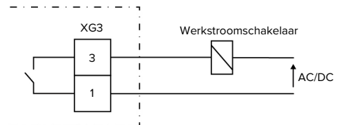
Afb. 10: Principe-schakelschema: Aansluiting van een externe werkstroomschakelaar
