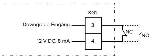
Abb. 14: Prinzipschaltbild: Anschluss eines externen Schaltkontakts (Standard-Einstellung: NO)
